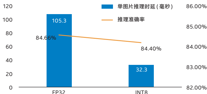
图二 腾讯云智能视频分析深度学习模型在不同计算精度下的推理准确率和速度比较
