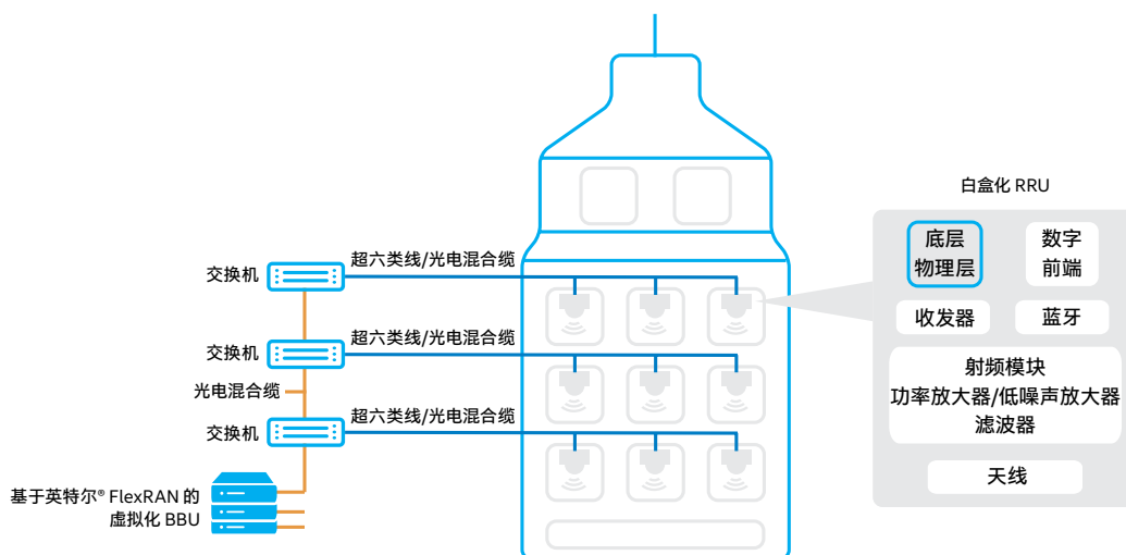
图一 新华三基于小基站的有源室分系统架构
