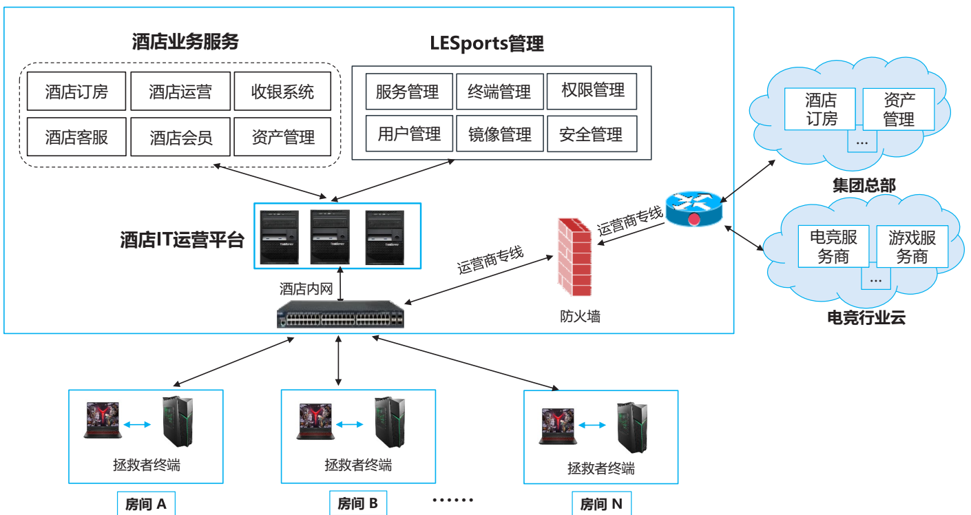
图 1. 联想电竞酒店云终端解决方案酒店拓扑图
